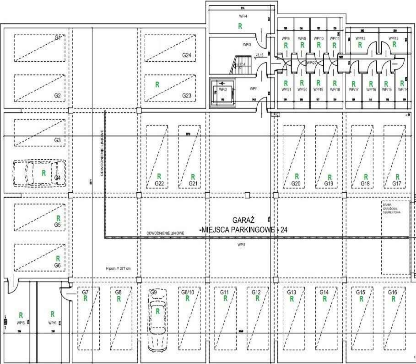
RZUT PIWNIC
