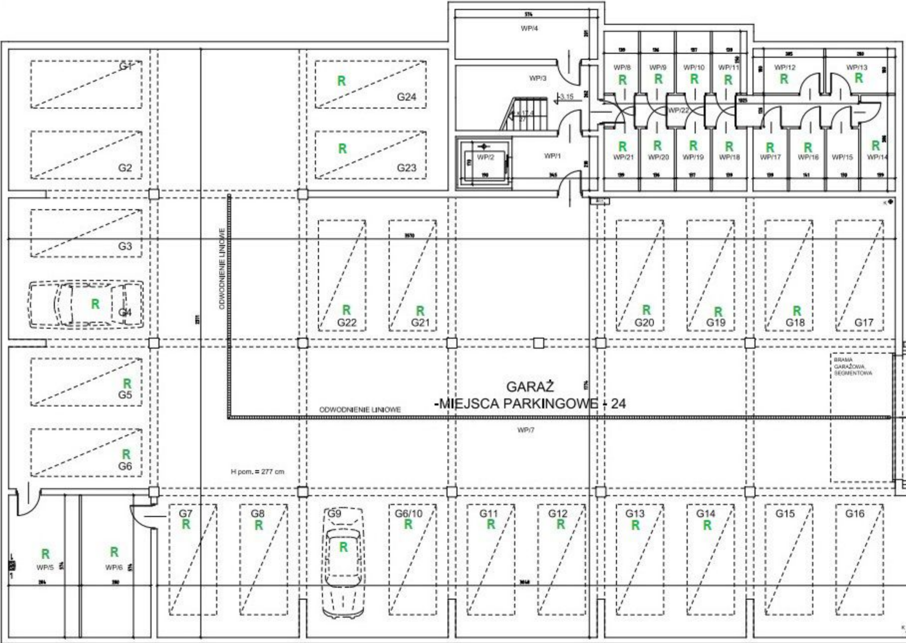
RZUT PIWNIC
